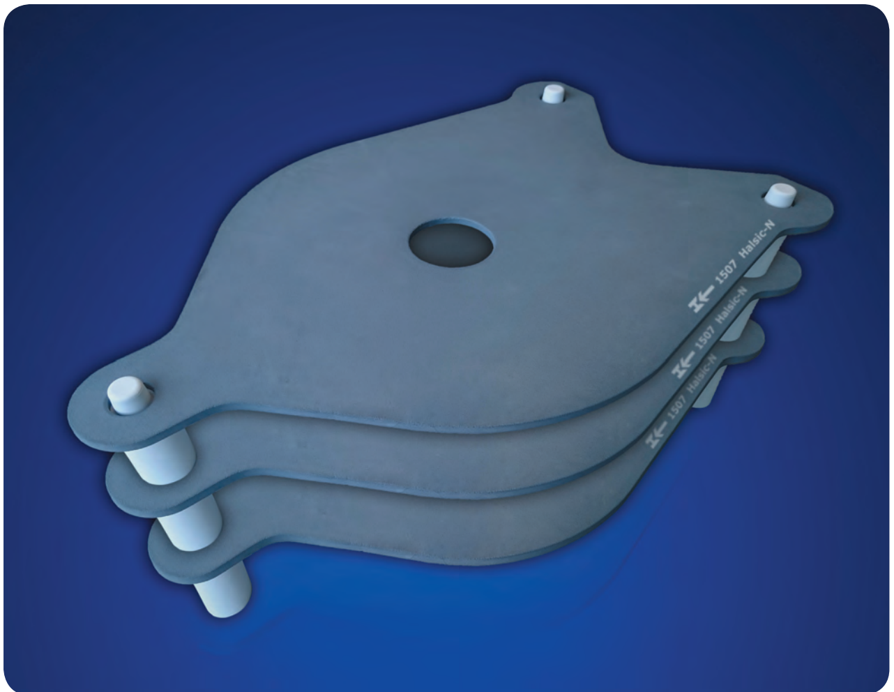
Typischer Brennhilfsmittelaufbau (Tellerständer) für den Einsatz in Porzellan-Schnellbrandöfen. Verschiedene Größen und Ausführungen sind je nach Kundenwunsch möglich.
